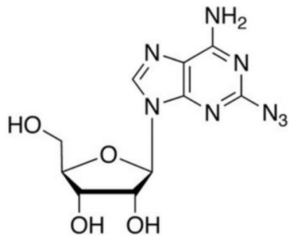
ADENOSINE
